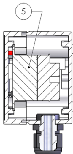
SEZIONE B-B
