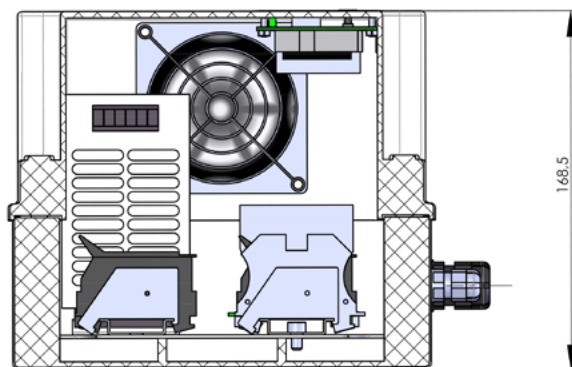
SEZIONE G-G
